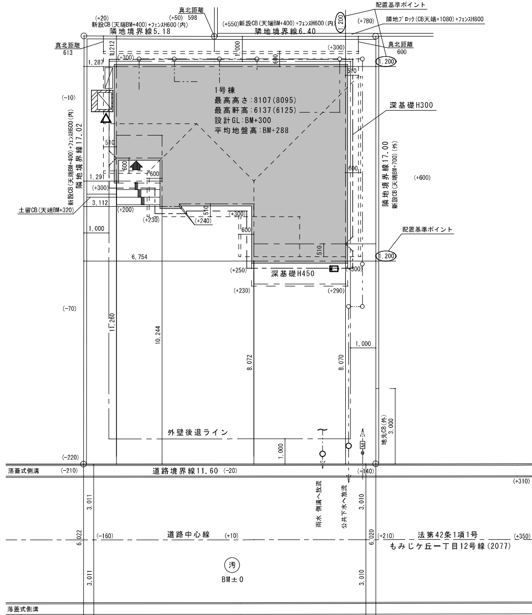
配置 図 S=1/100
